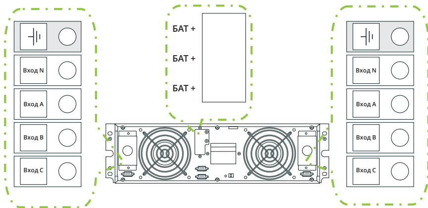
На рис. слева: Вход заземление/Вход нейтраль/Вход фаза A(L1), фаза B(L2), фаза C(L3) На рис. в середине: Положит. полюс батарей/Общий батарей/Отрицат. полюс батарей На рис. справа: Выход заземление/Выход нейтраль/ Выход фаза A(L1), фаза B(L2), фаза C(L3)
